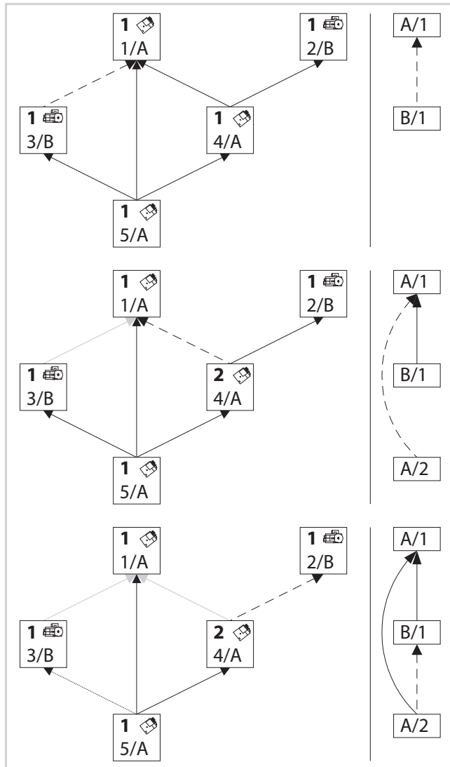
Bild D.12: Verfahren zur Erzeugung eines zyklensfreien Ressourcen-Graphen (Teil 1)
