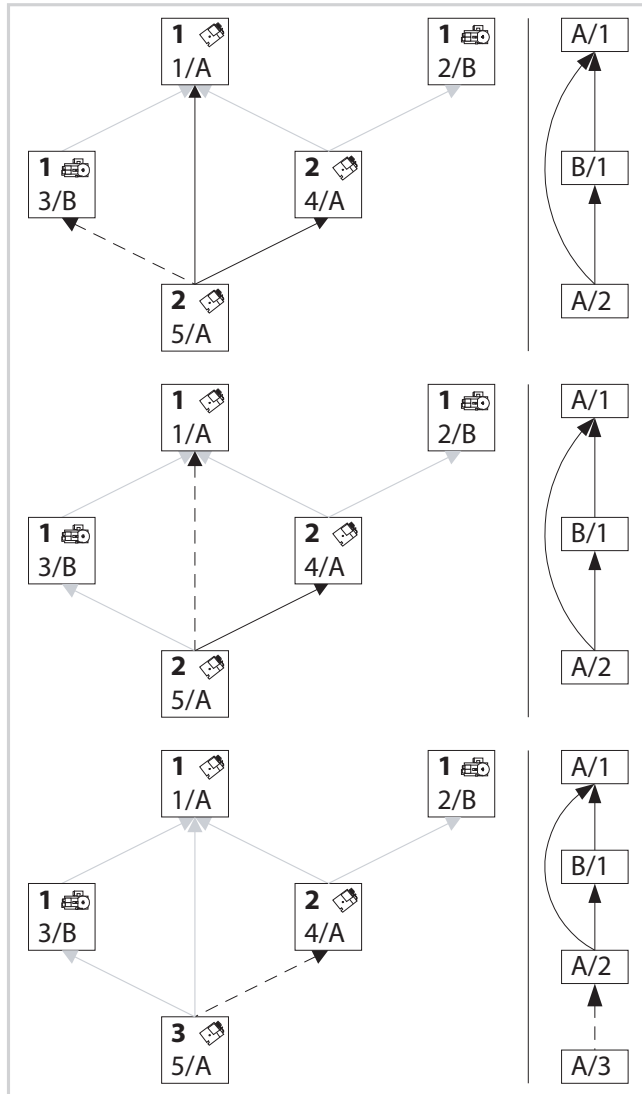
Bild D.13: Verfahren zur Erzeugung eines zyklensfreien Ressourcen-Graphen (Teil 2)
